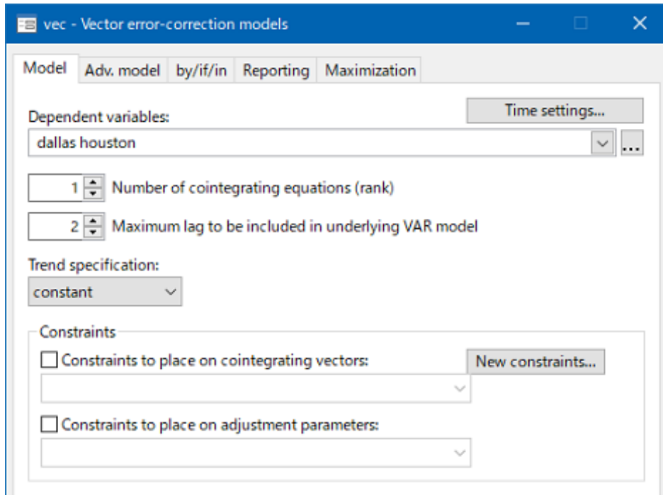
図 5 vec ダイアログ - Model タブ
