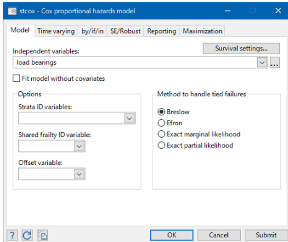
図2 stcox ダイアログ- Model タブ
