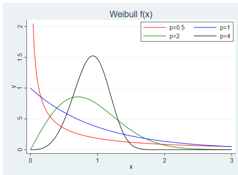
図1 Weibull 分布の確率密度関数
